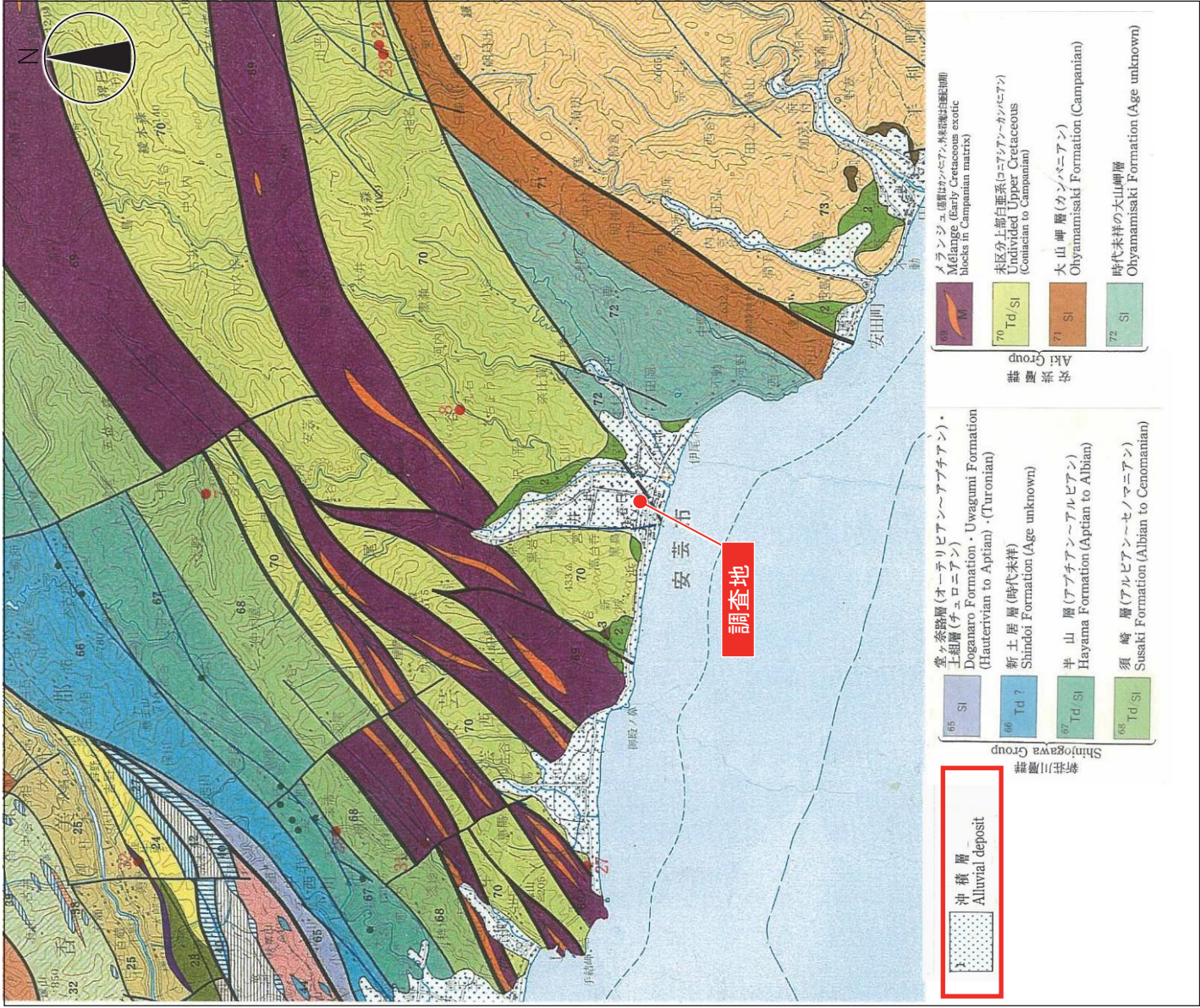
図 1-2 調査地周辺の地質
