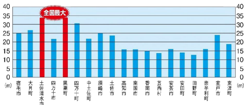
海岸線での津波の高さ
