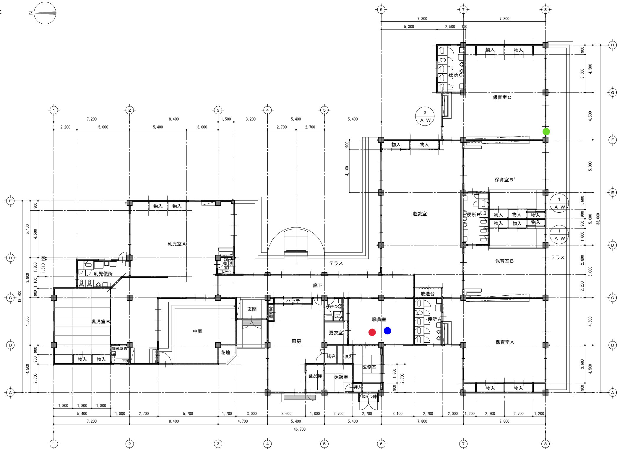
1 階平面図
