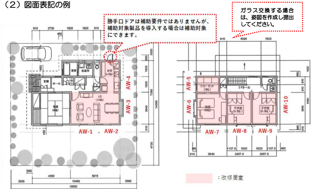
図9 窓改修寸法
