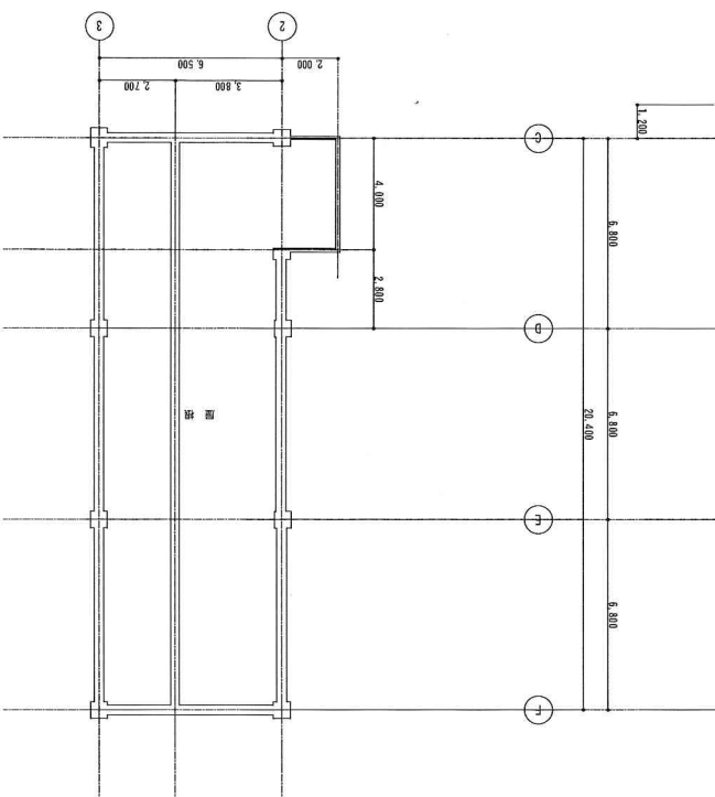
屋顶平面图
