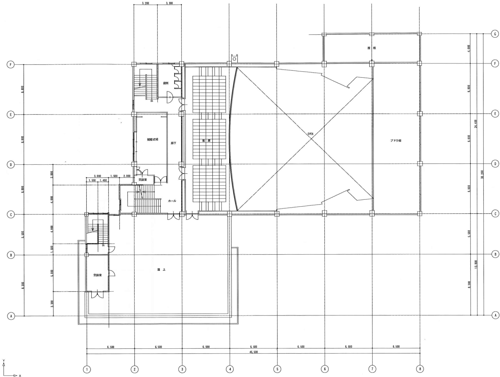
3階平面図
