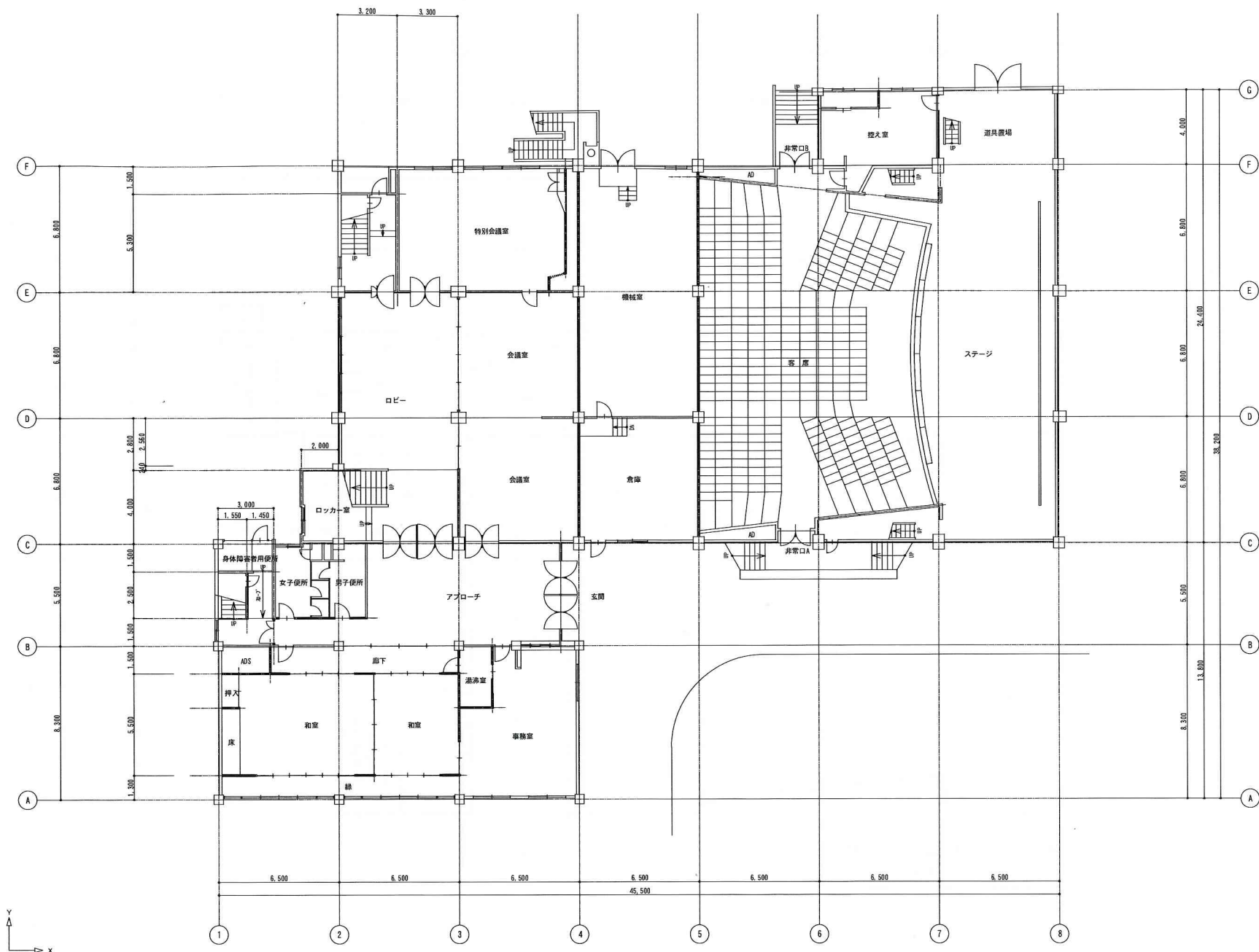
1階平面図
