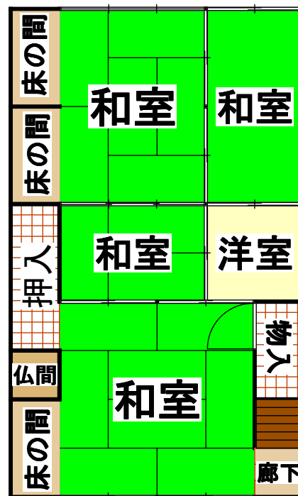
2F平面図
