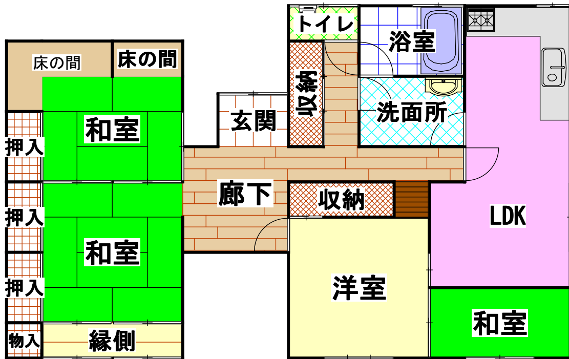
1F平面図
