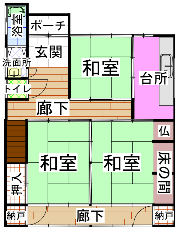
1F平面図
